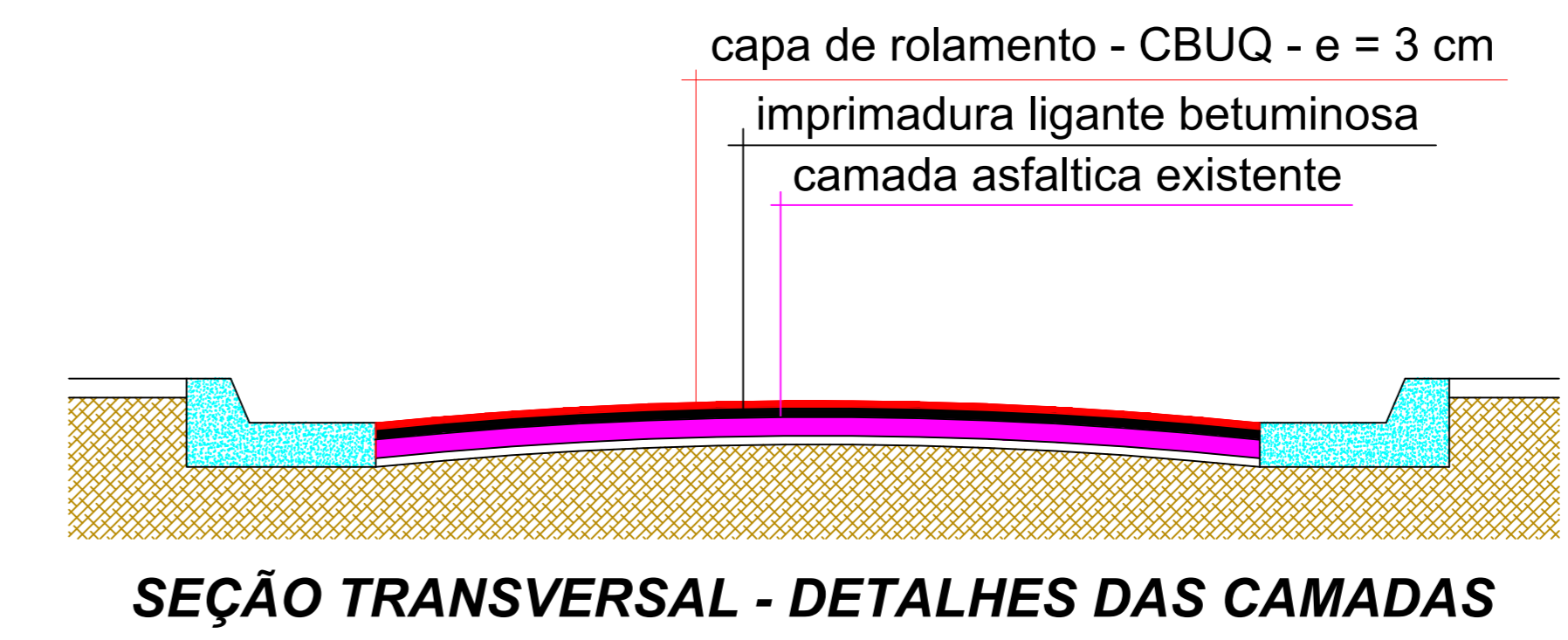
Detalhe 01 - Recapeamento Asfáltico (CBUQ)
