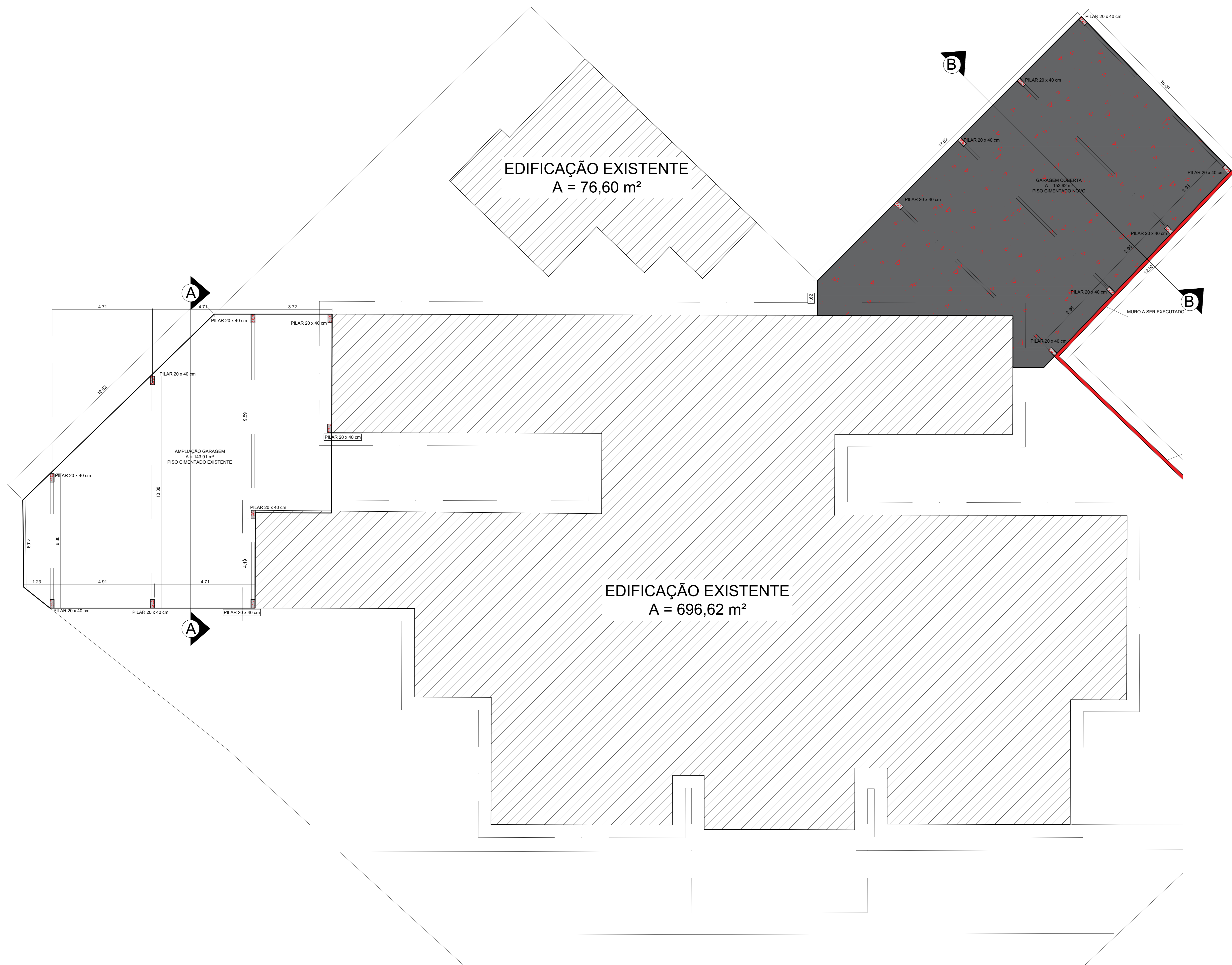
PLANTA BAIXA – AMPLIAÇÃO ESCALA 1:100
